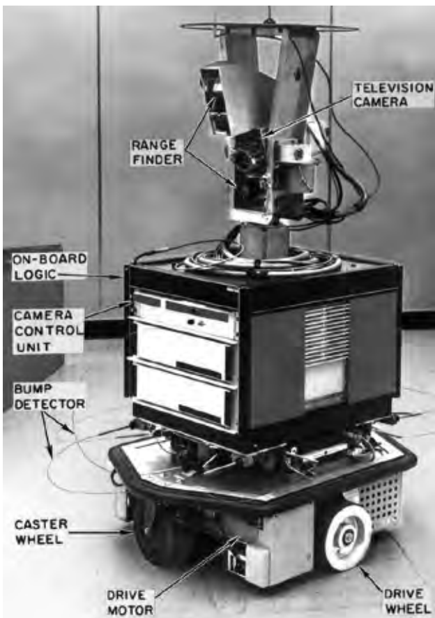
Abbildung 1.(a) Kognitiver Roboter Shakey (Quelle: SRI AI Center).
