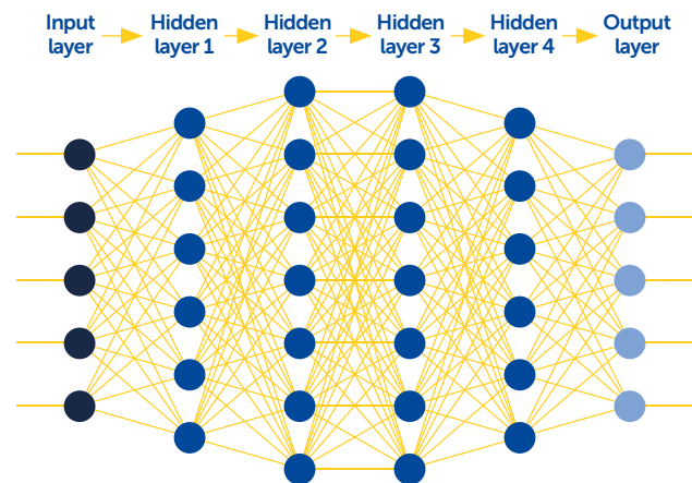
Abbildung 1.(b) Beispiel für tiefes neuronales Netz 15 .
